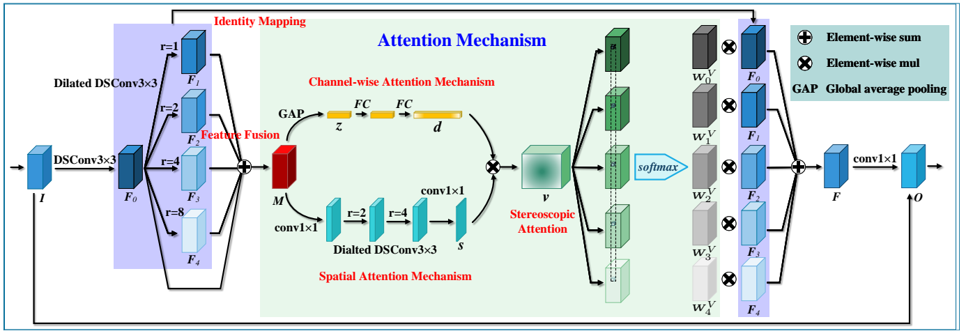
图 1. 对我们提出的 SAM 模块的图示。给出输入特征图像 I 的情况下, SAM 首先会通过多个分支来提取多尺度的特征 F_i (i = 0, 1, \dots, N) 。多尺度特征 F_i 会通过逐元素相加的方法整合并得到 M 。然后, 我们基于 M 计算逐通道的注意力 logits d 以及空间注意力 logits s 。把 d 和 s 相乘获得空间注意力 logits v , 然后使用 \text{softmax} 函数来获得空间注意力权重 w_i^v (i = 0, 1, \dots, N) 。 w_i^v (i = 0, 1, \dots, N) 是被用于整合 F_i 为 F 的权重。最后, 一条残差连接 [43] 从 I 连接到最后并相加获得输出 O 。图中, \otimes 表示逐元素乘法, 并且两个相乘的特征图像会在相乘前复制为同样的形状。符号 r 表示膨胀卷积 3 \times 3 膨胀卷积的膨胀率。在彩色下观看以获得最好效果。
